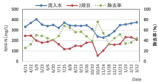
図7 NH 4 -Nの濃度と除去率の変化
